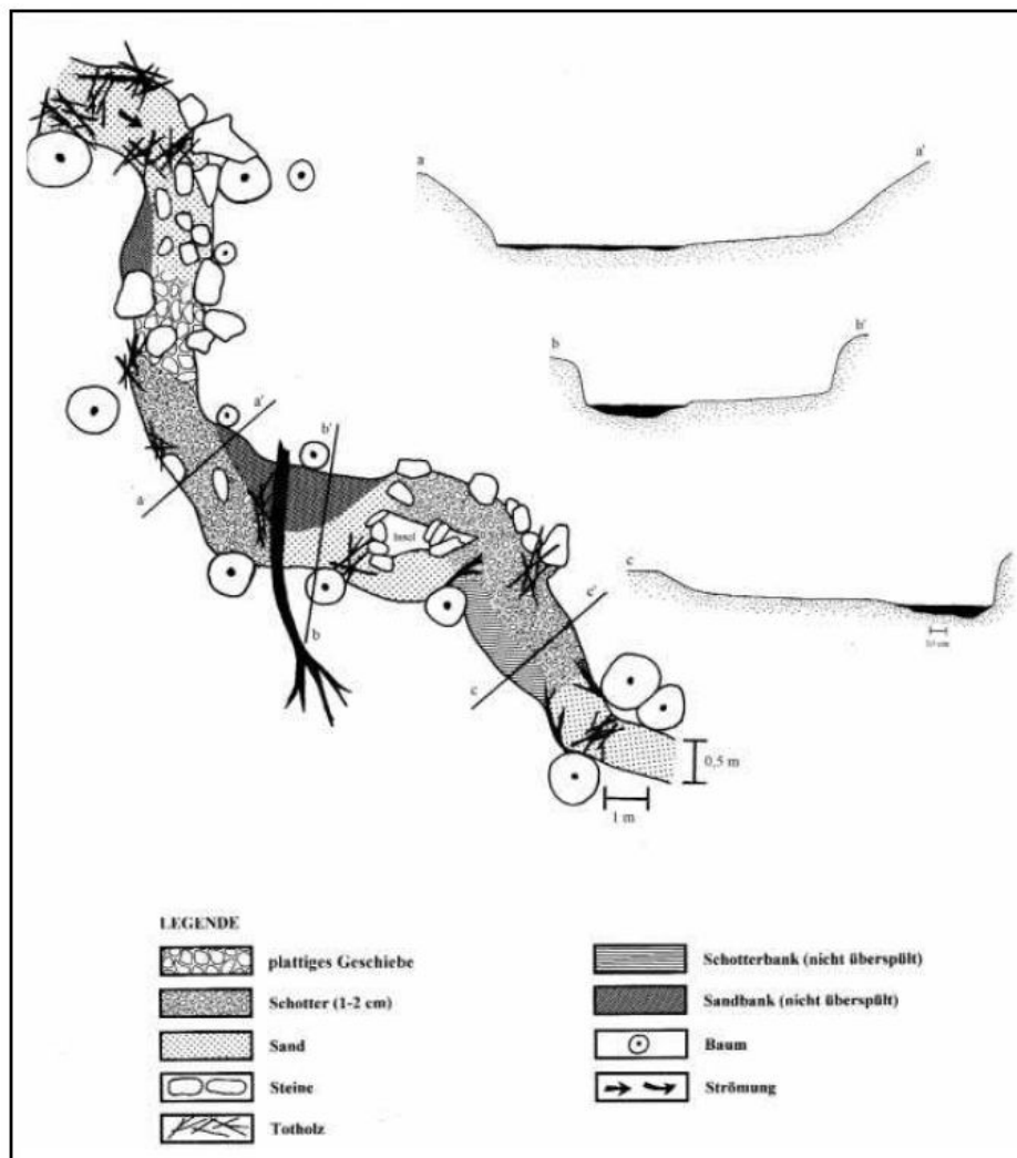
Abbildung 1: Beispiel für die Verteilung der Substrate auf der Bachsohle und die Querprofilausbildung eines Kleinen Talauebaches im Deckgebirge (LUA 1999)
